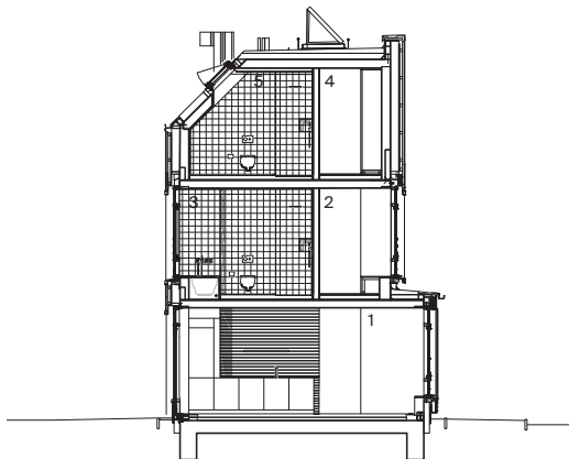
1 Wohnküche 2 Sonnendiele 3 Bad 4 Flur 5 Bad
