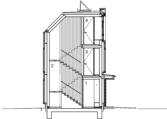
1 Garderobe 2 Treppenhaus 3 Flur 4 Sonnenplatz
